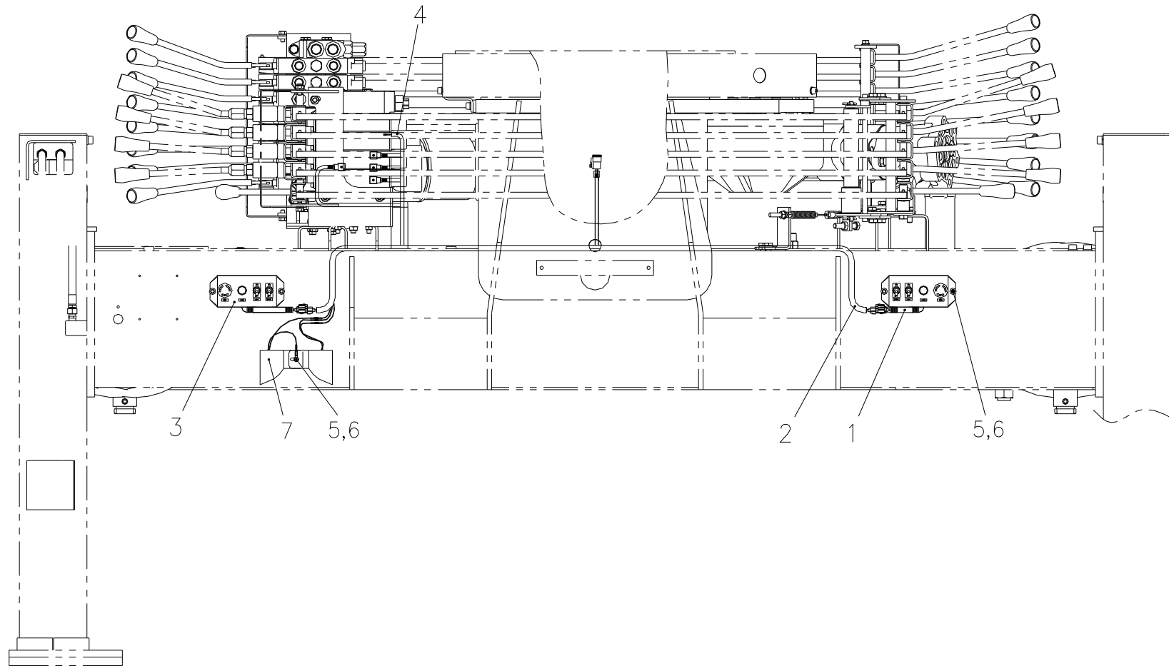
프레임 전선 Fig. 9-1 SCS506 FRAME WIRING
