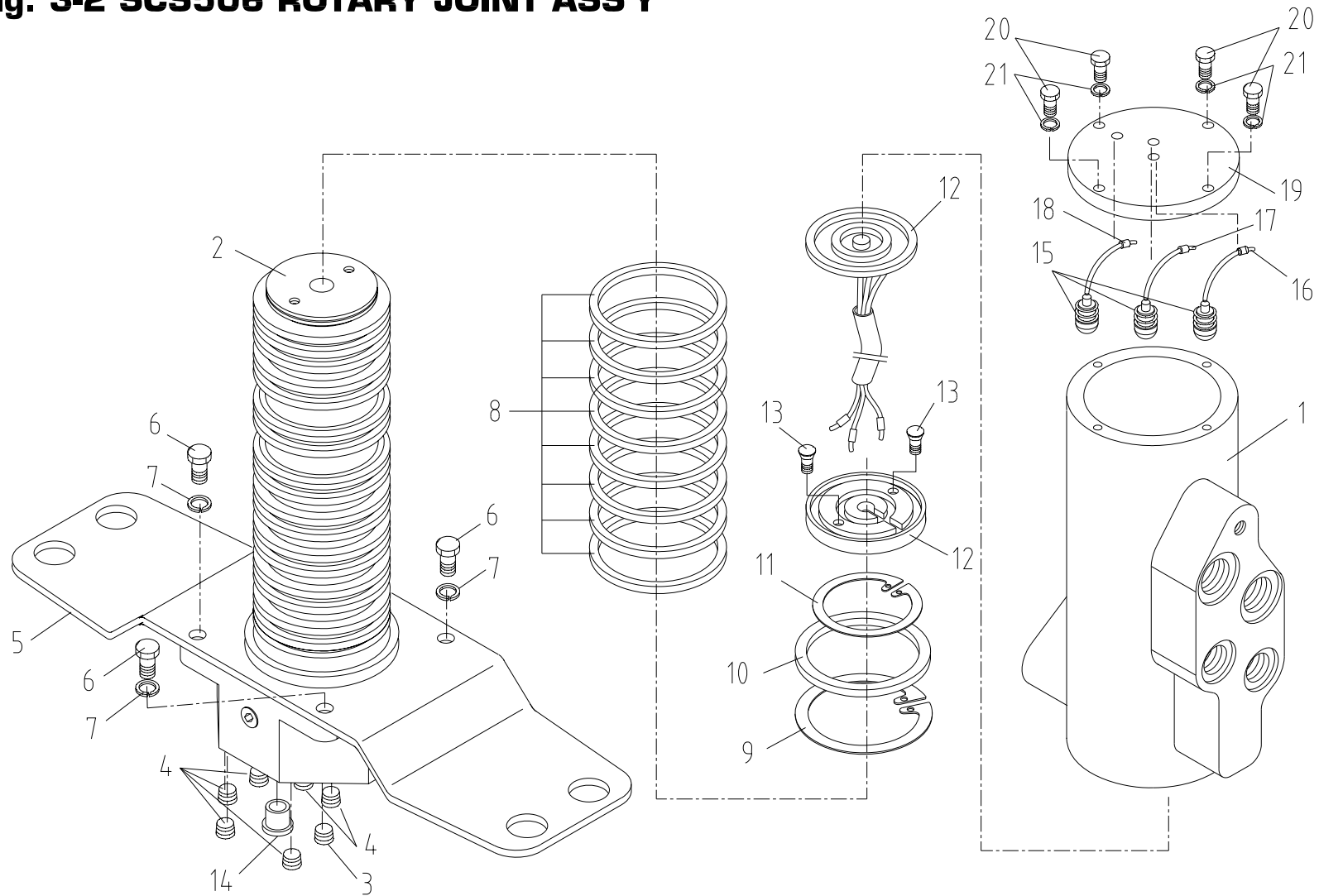
로타리 조인트 조립체 Fig. 3-2 SCS506 ROTARY JOINT ASS'Y
