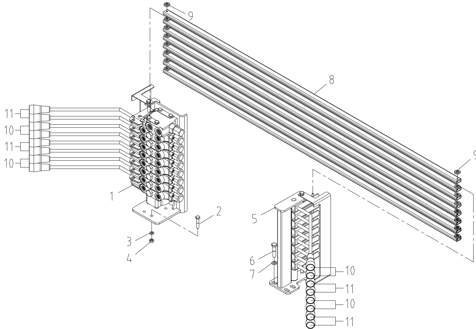
오퍼레이션 아우트리거 조립체 Fig. 3-4 SCS506 OPERATION OUTRIGGER ASS'Y
