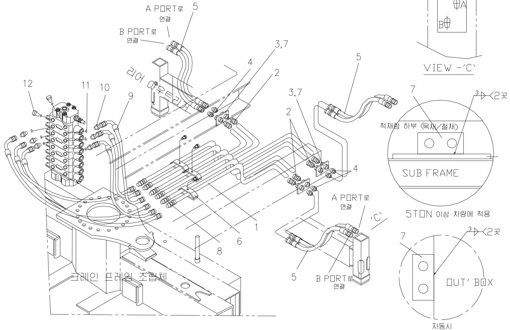
장착 배관 파트(5Ton) Fig. 8-5 SCS506 R/ A M/ T PIPING PART(5Ton)
