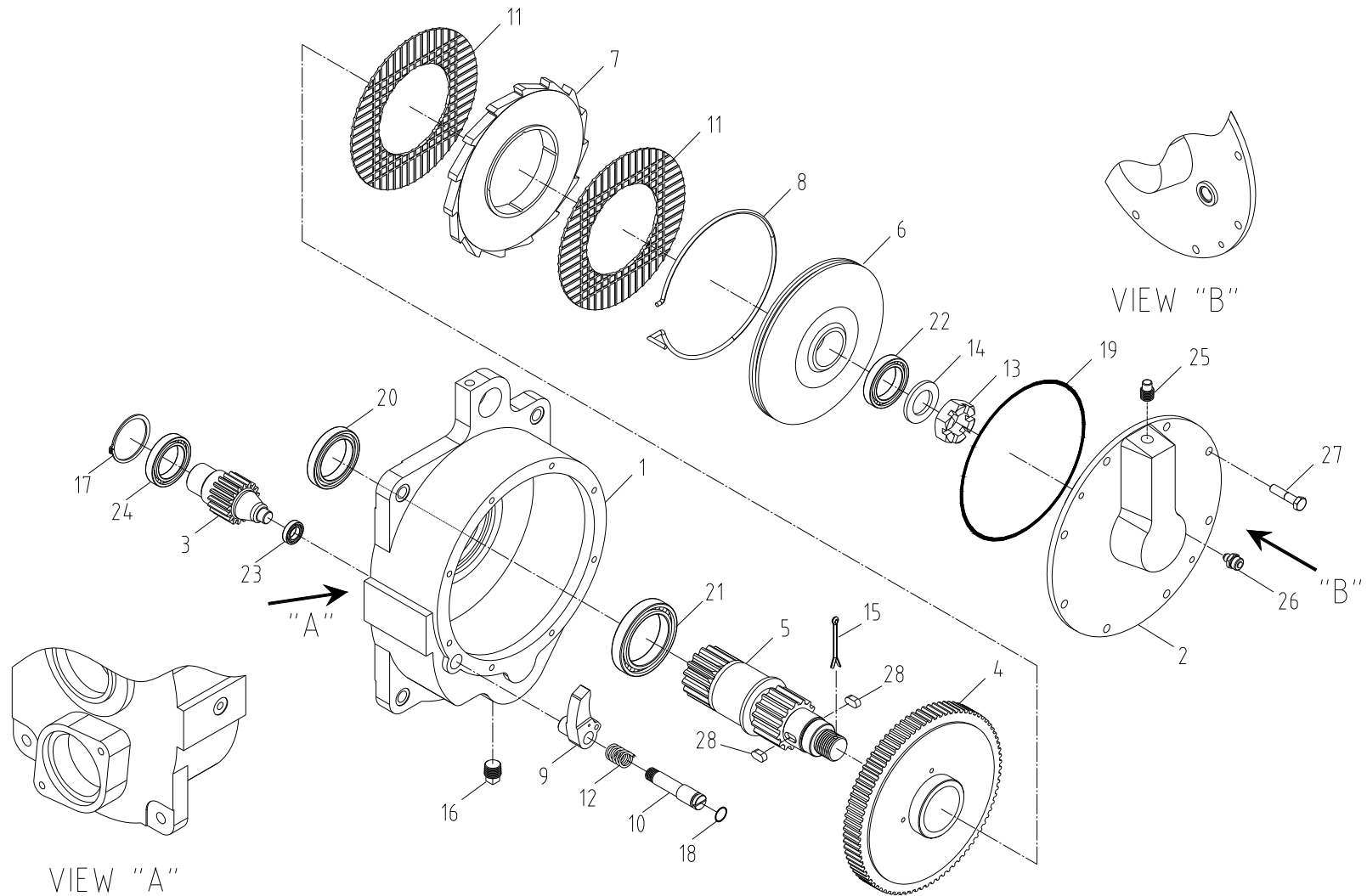
원치 감속기 조립체 Fig. 2-1 SCS506 WINCH R/ G ASS'Y
