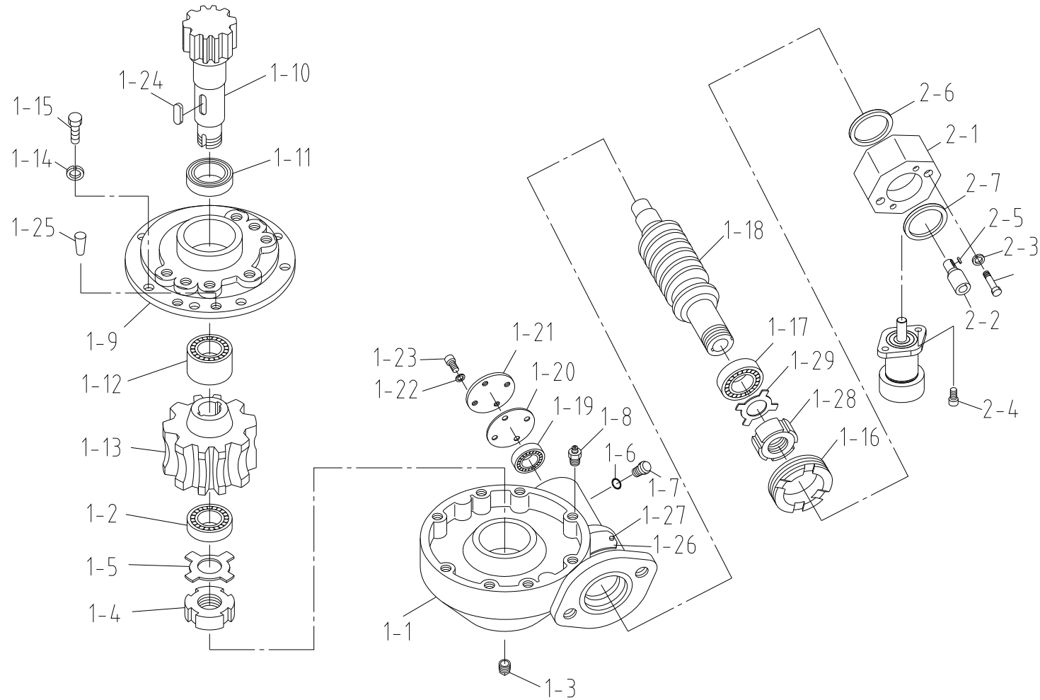
스윙 감속기 세트 Fig. 3-1 SCS506 SWING R/ G SET
