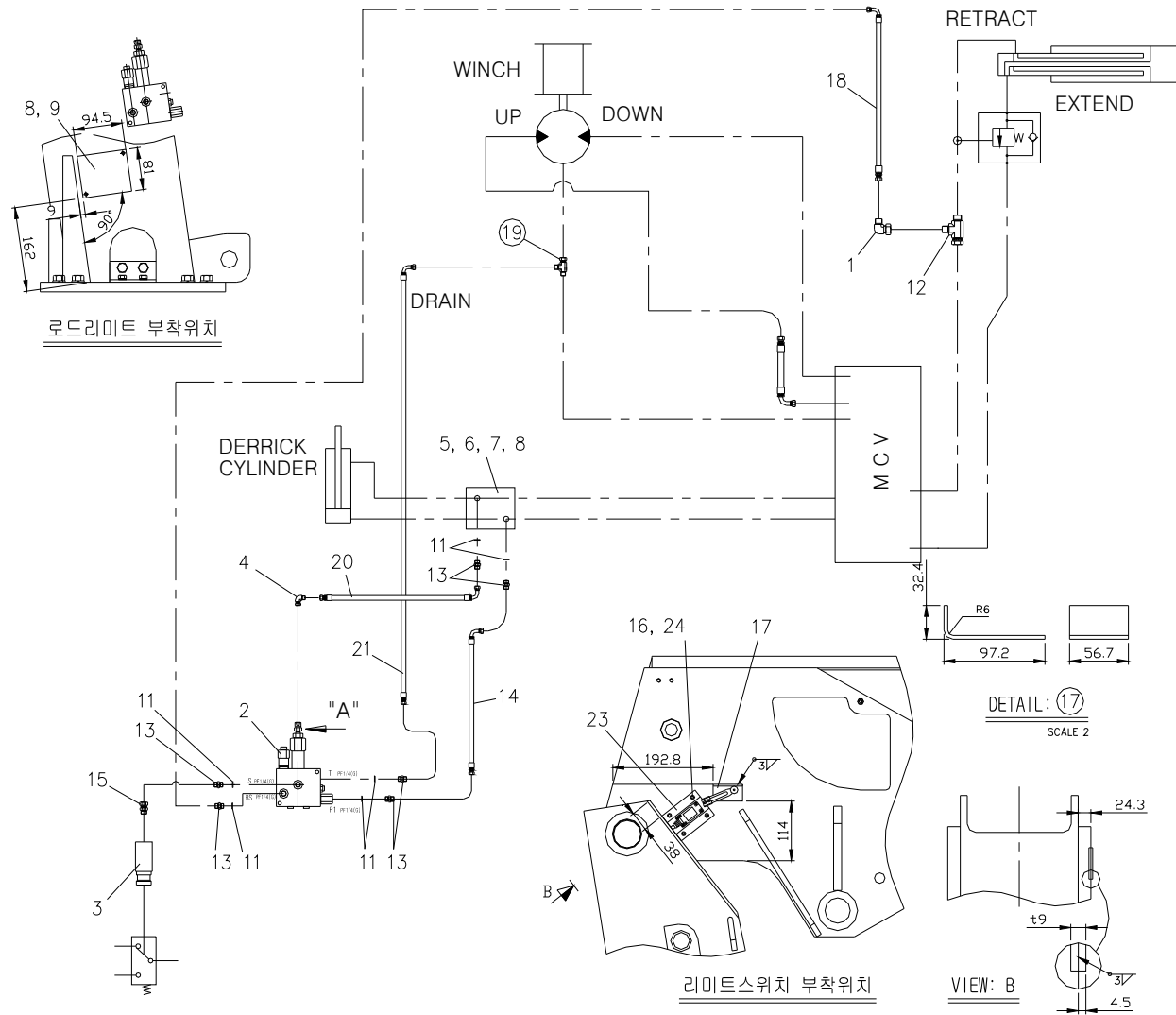
Fig. 11 SCS506 과하중 방지 PIPING ASS'Y
