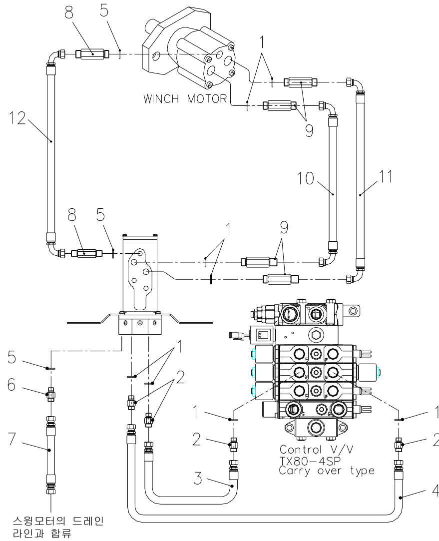
메인 윈치 배관 Fig. 5-3 SCS506 MAIN WINCH PIPING
