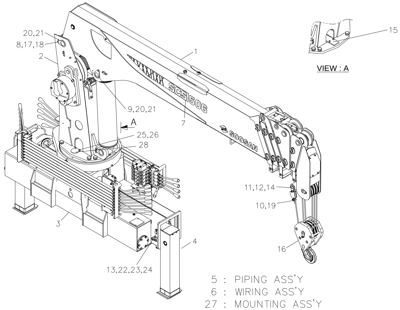
크레인 조립체 Fig. 0 SCS506 CRANE ASS'Y
