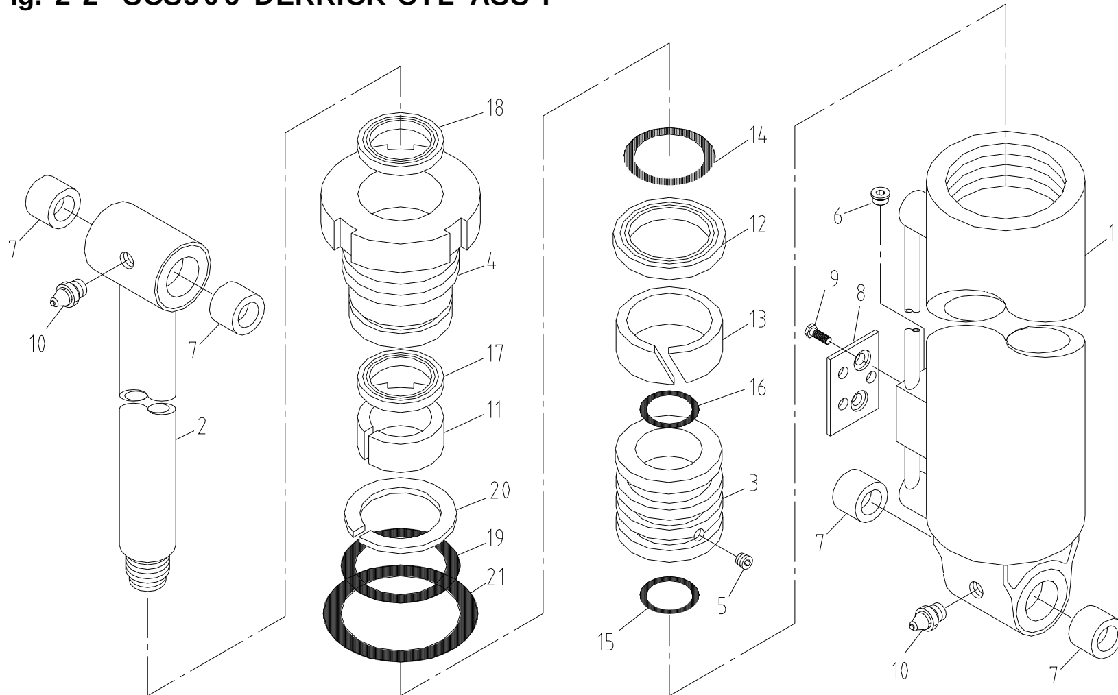
데릭 실린더 조립체 Fig. 2-2 SCS506 DERRICK CYL' ASS'Y
