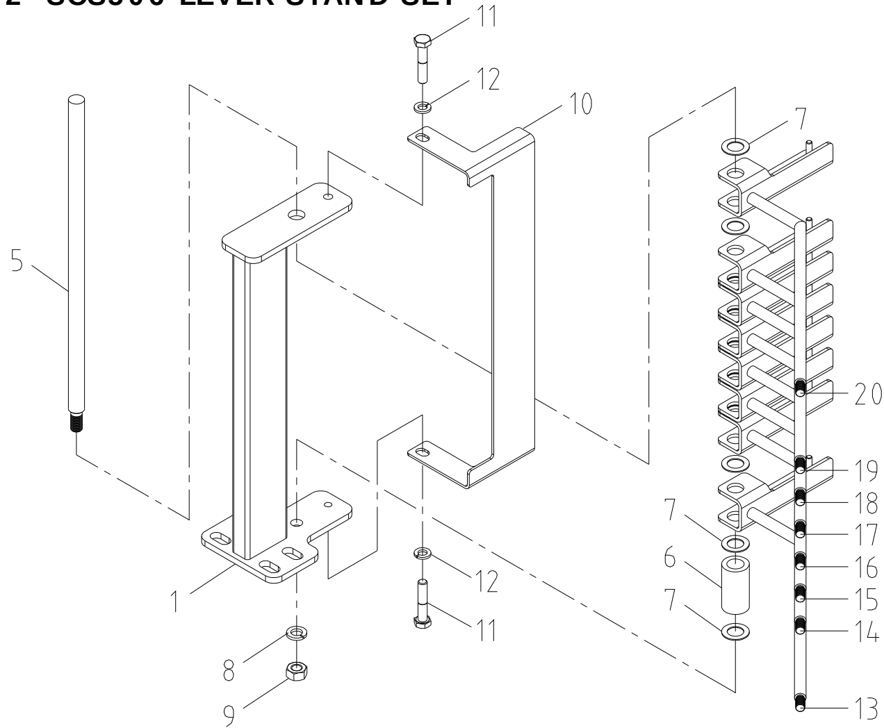
레버 스텐드 셋 Fig. 3-4-2 SCS506 LEVER STAND SET
