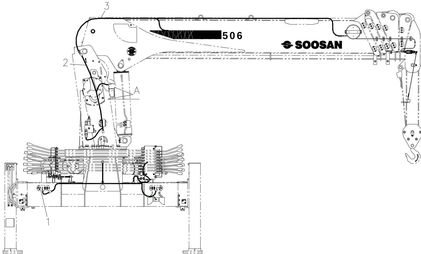
전선 조립체 Fig. 9 SCS506 WIRING ASS'Y
