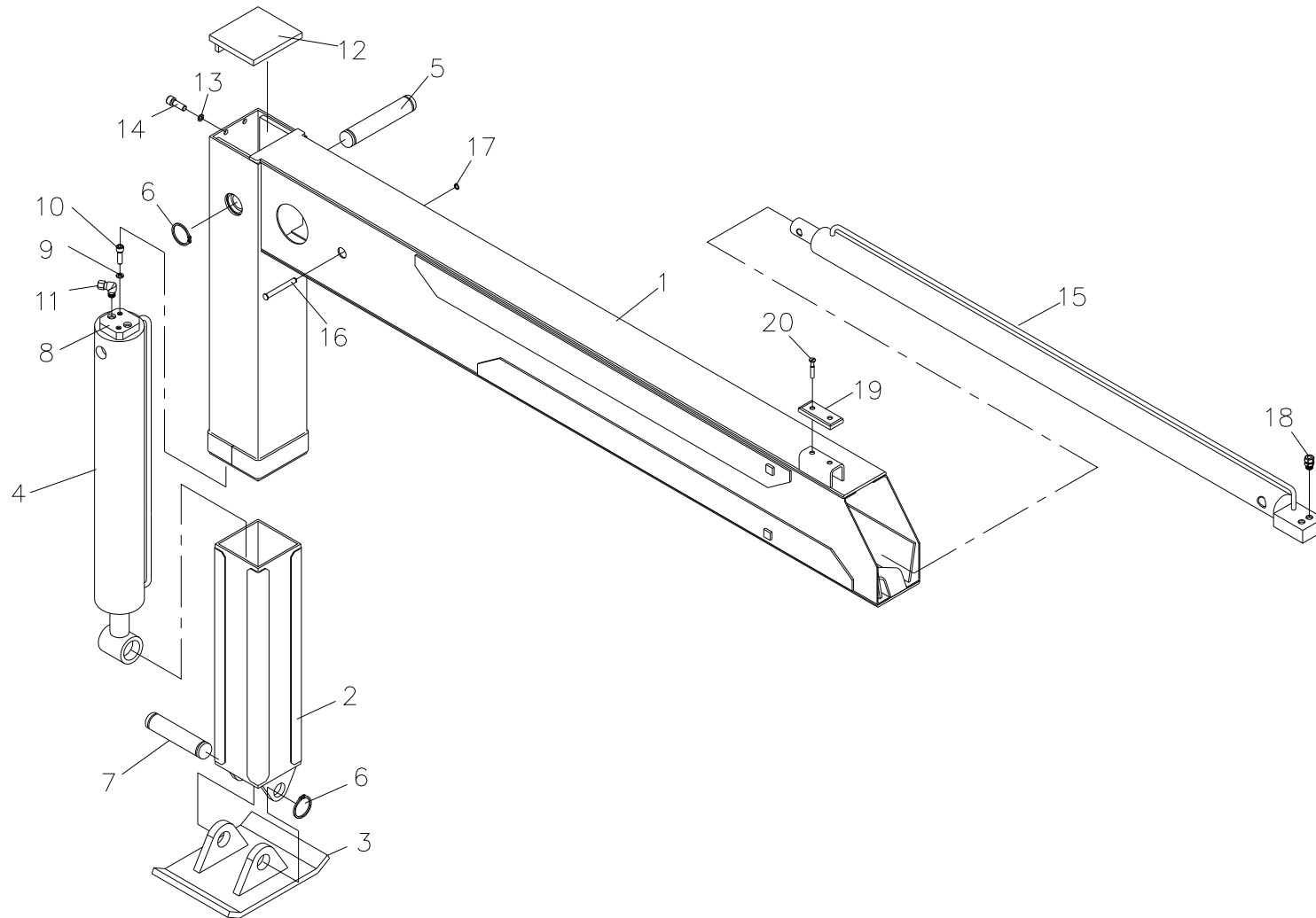
아우트리거 조립체 Fig. 4 SCS506 OUTRIGGER ASS'Y
