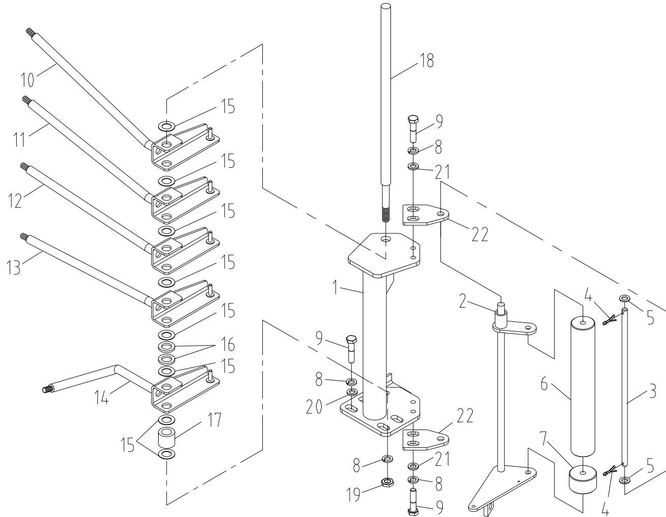
레버 스텐드 셋 Fig. 3-3-2 SCS506 LEVER STAND SET
