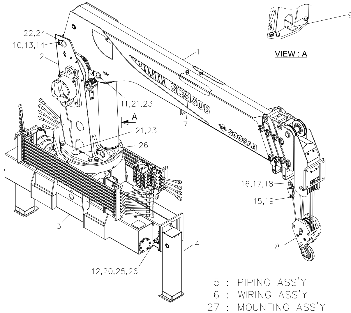
크레인 조립체 Fig. 0 SCS505 CRANE ASS'Y
