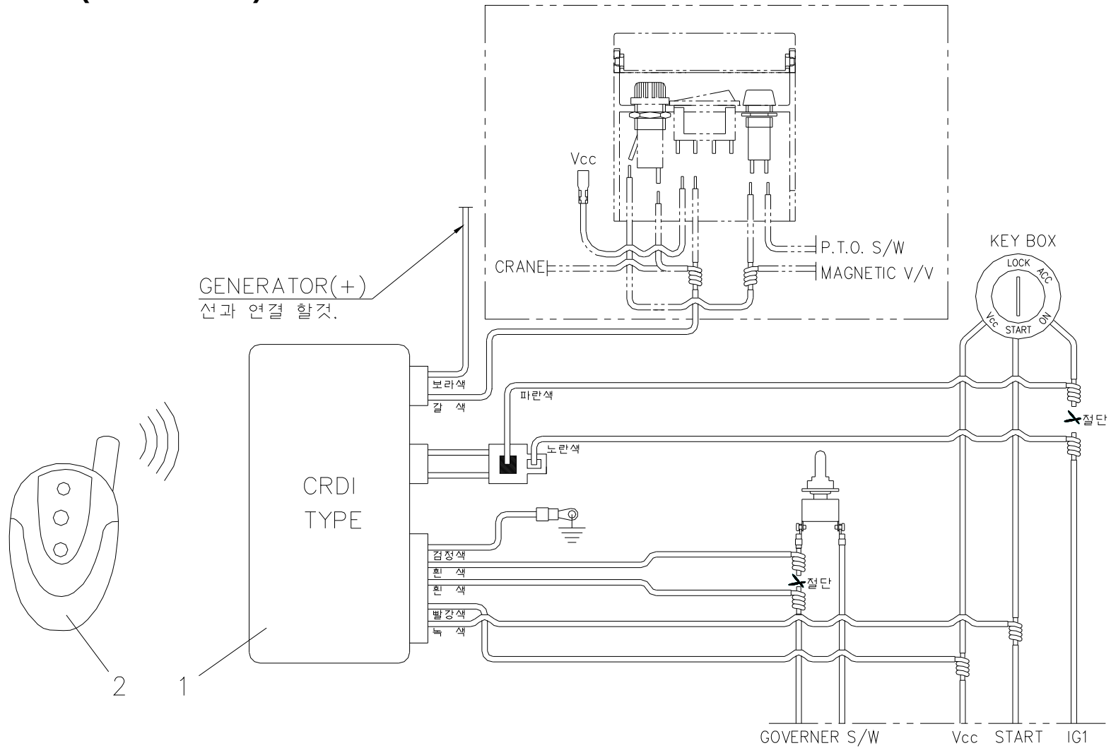
Fig. 12 SCS506 무선 상부 시동 장치 SET (CRDI TYPE)
