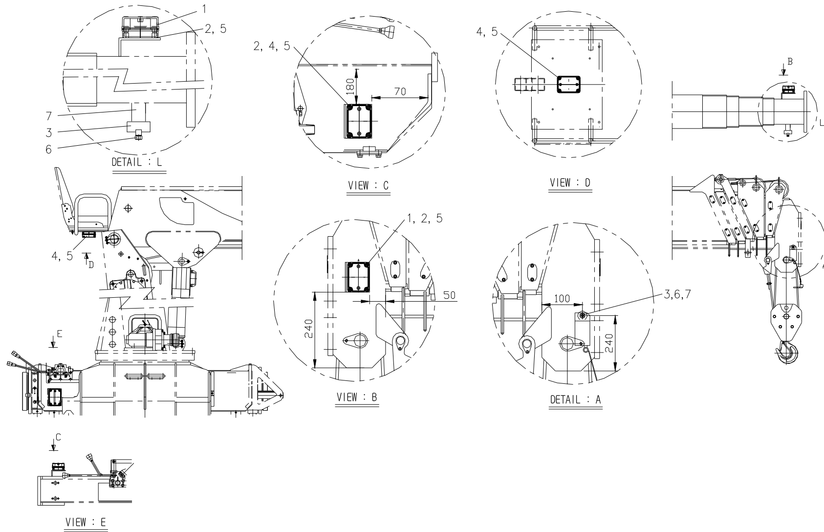
Fig. 10 SCS506 무선과권 장치 위치도
