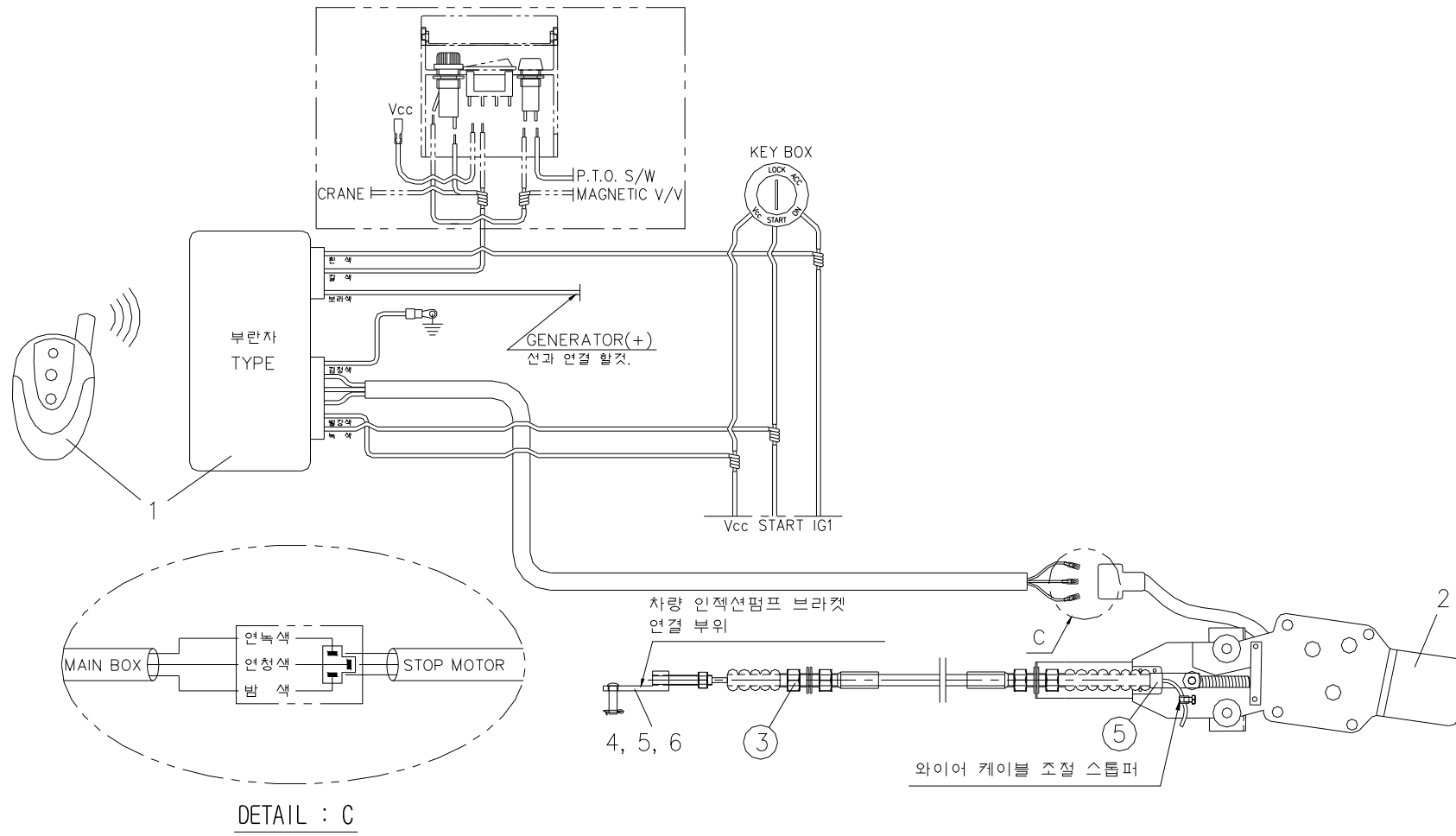
Fig. 13 SCS506 무선 상부 시동 장치 SET (부란자 TYPE)
