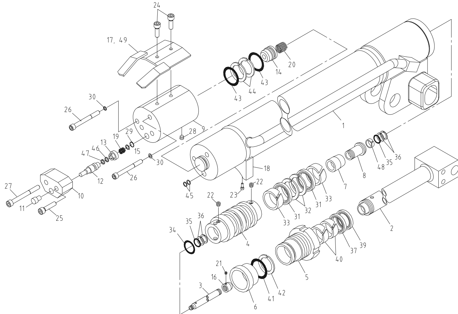
텔레스코픽 실린더(1단) 조립체 Fig. 1-1-1 SCS506 TELESCOPIC CYL'(1st) ASS'Y
