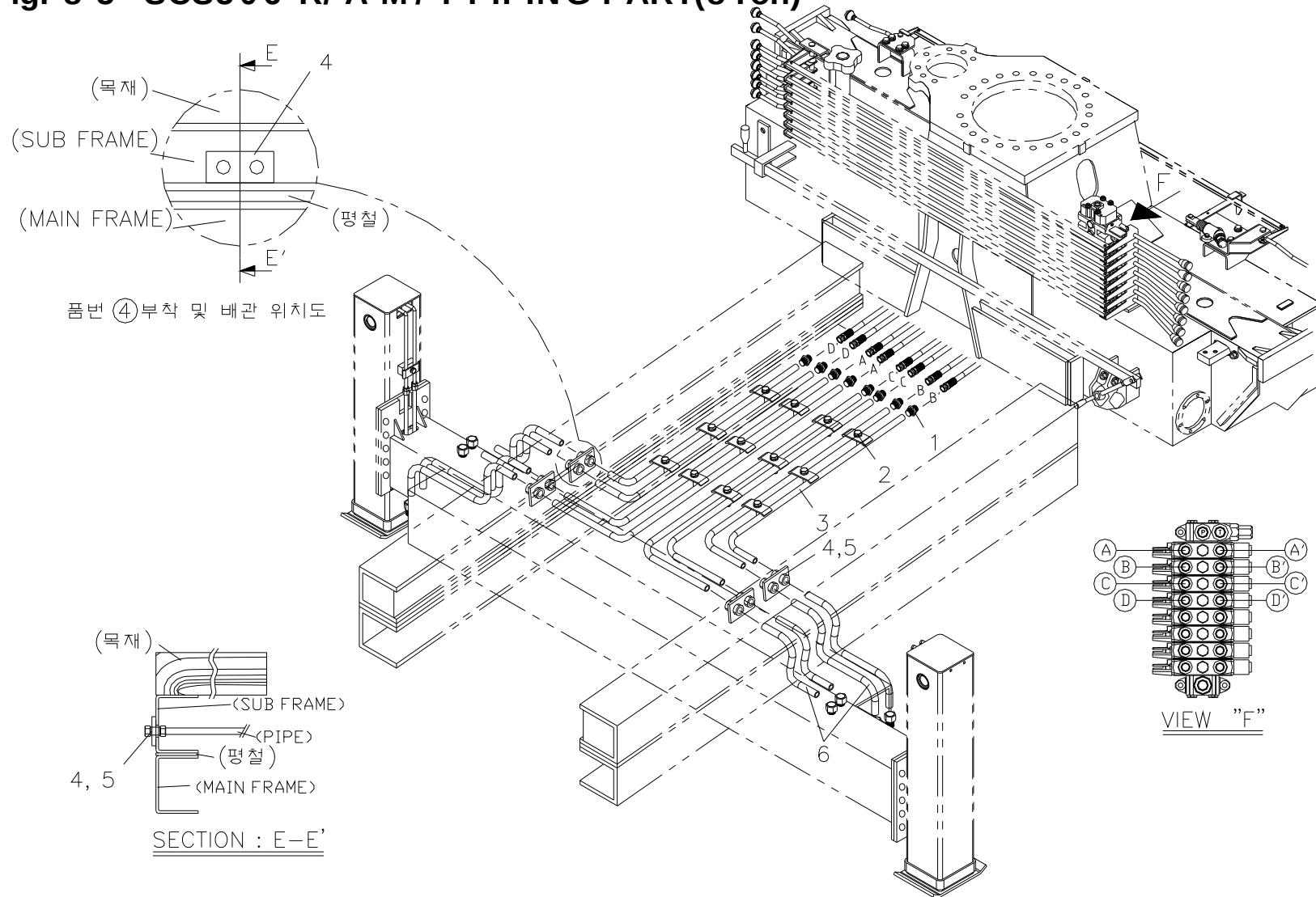
장착 배관 파트(8Ton) Fig. 8-5 SCS506 R/ A M/ T PIPING PART(8Ton)
