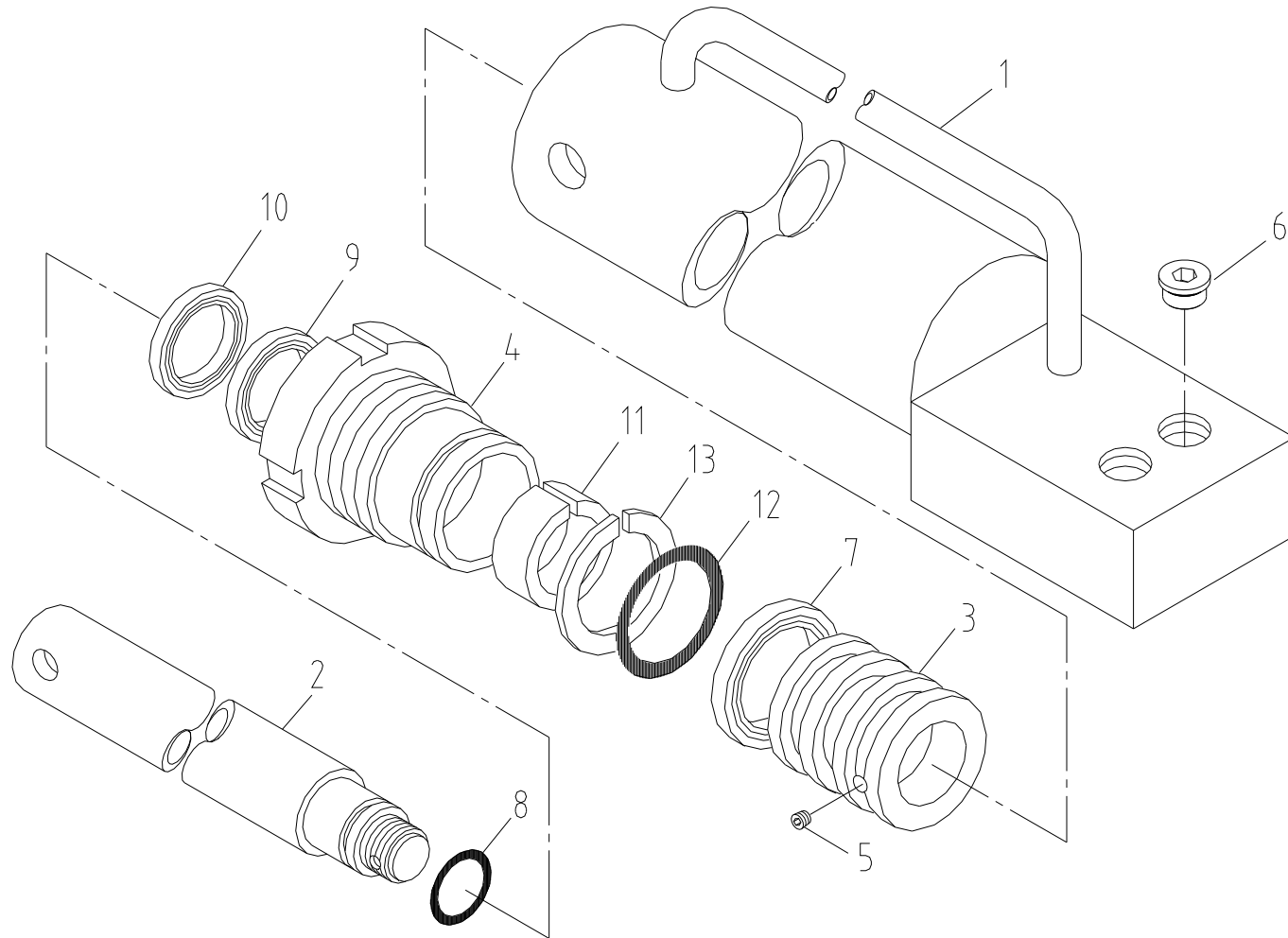
익스펜드 실린더 조립체 Fig. 4-2 SCS506 EXPAND CYL' ASS'Y
