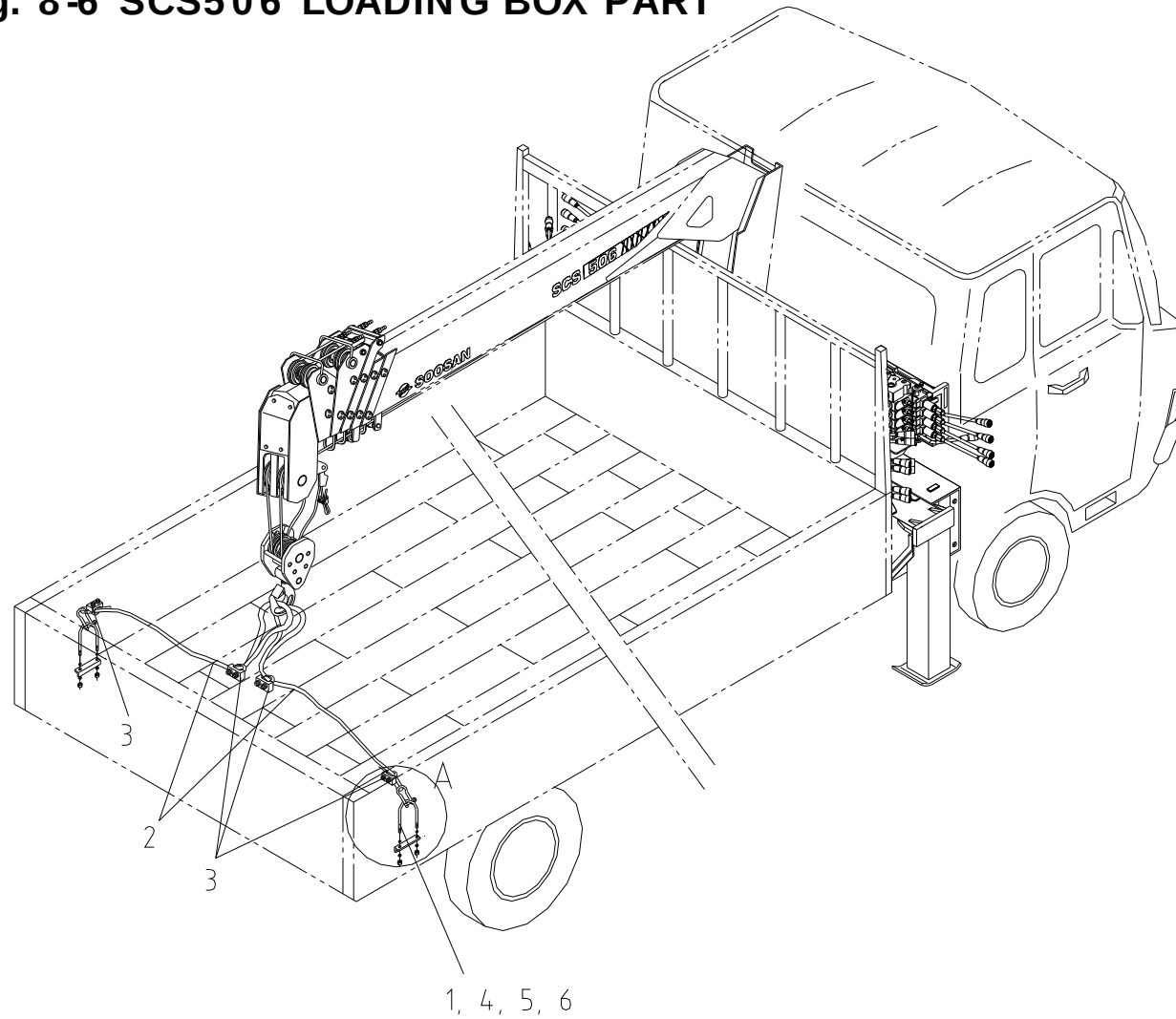
로딩 박스 파트 Fig. 8-6 SCS506 LOADING BOX PART
