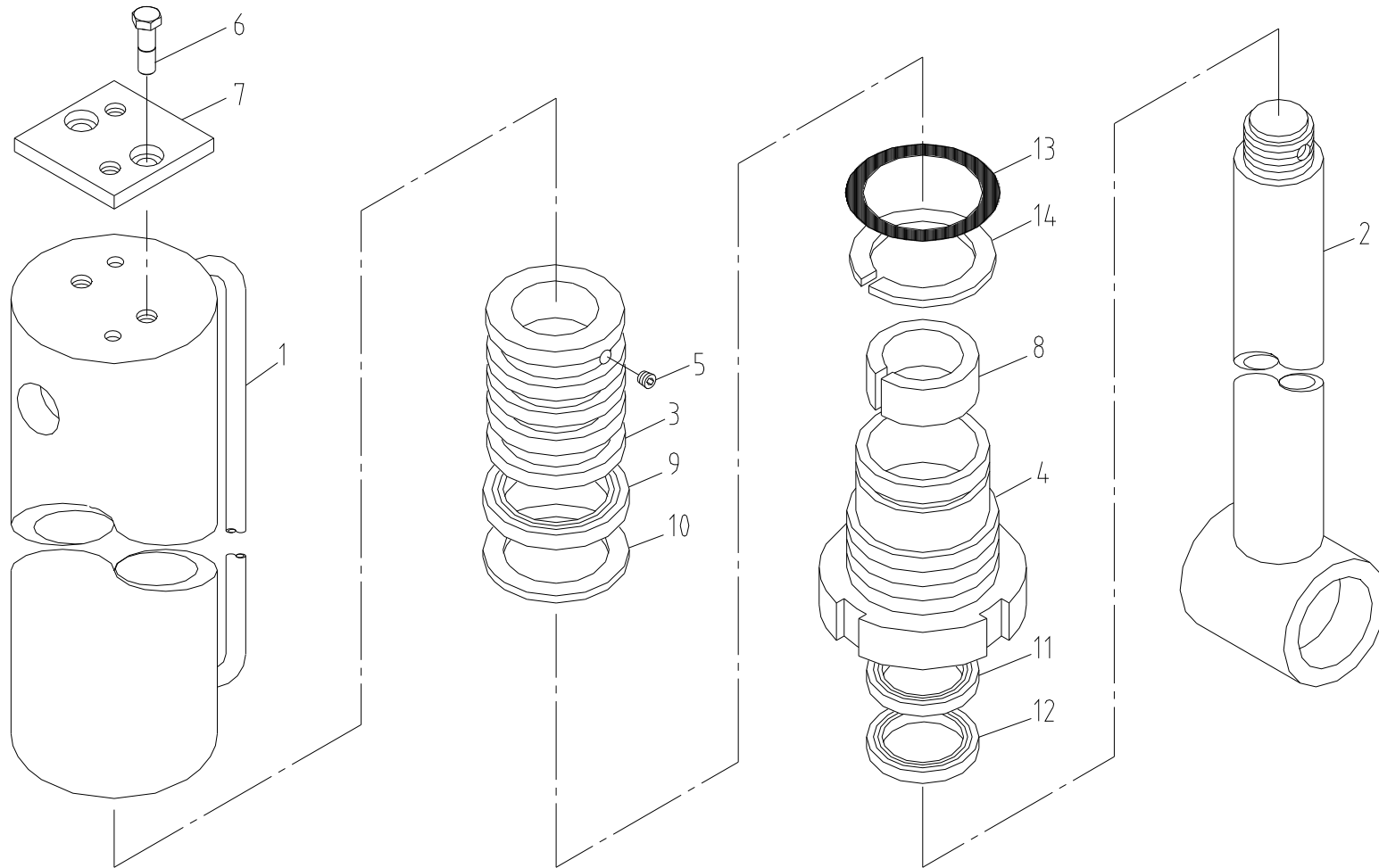
잭 실린더 조립체 Fig. 4-1 SCS506 JACK CYL' ASS'Y
